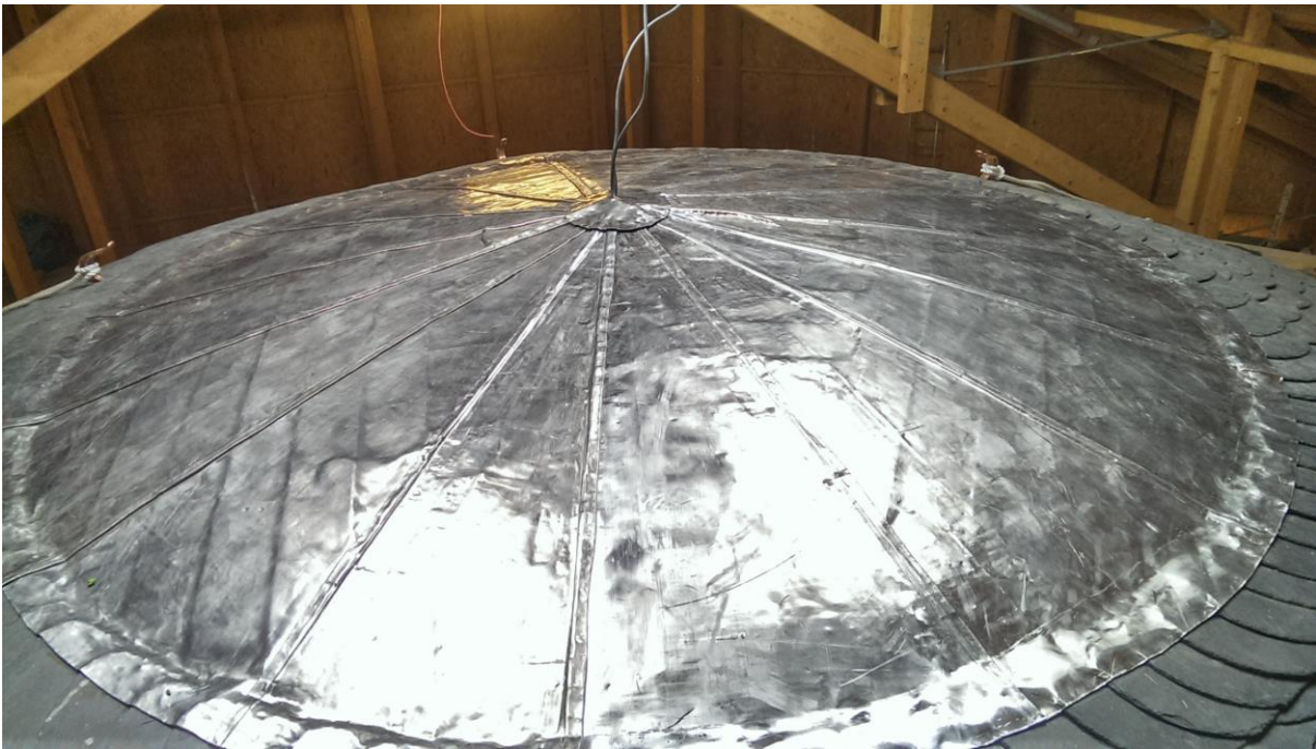
Abb. 19: Die gesamte Bleieindeckung setzt sich zusammen aus 15 Kreissektoren.
